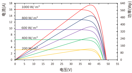
不同辐照度下, I-V 曲线图
